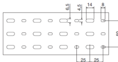
T1-ZH Largeurs 80 100 et 120 mm Perforations du socle
