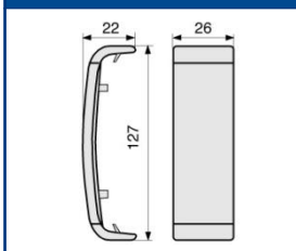
GBA Joint de couvercle
