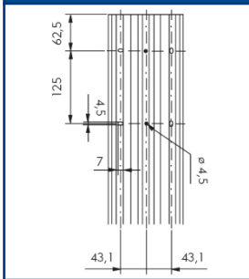
TBA Plinthes et Chambranles
