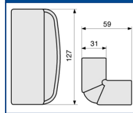
AEBA Angle extérieur variable
