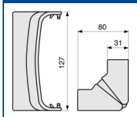
AIBA Angle intérieur variable
